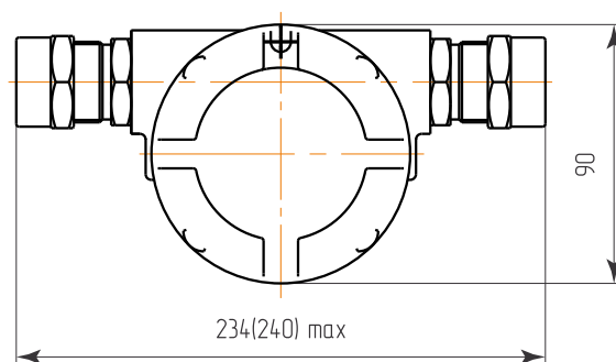
с двумя кабельными вводами
