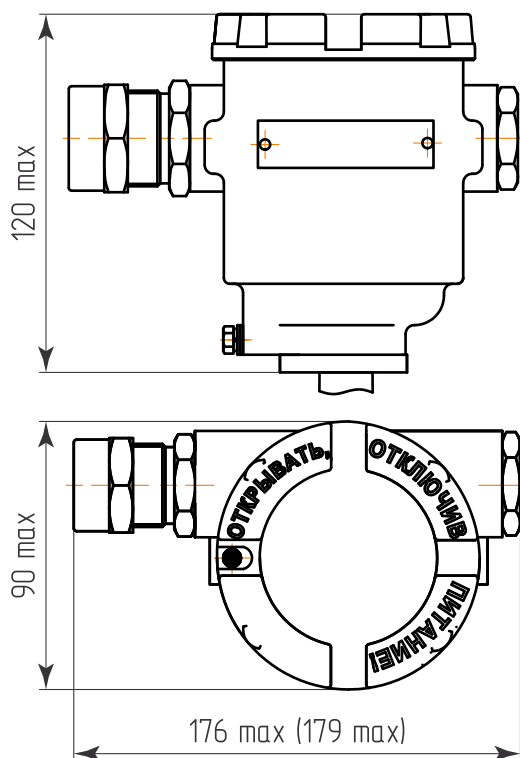
с одним кабельным вводом
