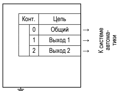
схема подключения выходов с нормально замкнутым (НЗ) или нормально разомкнутым (НР) состоянием
