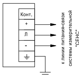
интерфейс СЕНС
