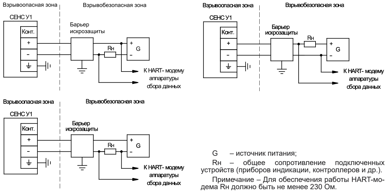
Схема подключения к системе с интерфейсом 4-20 мА
