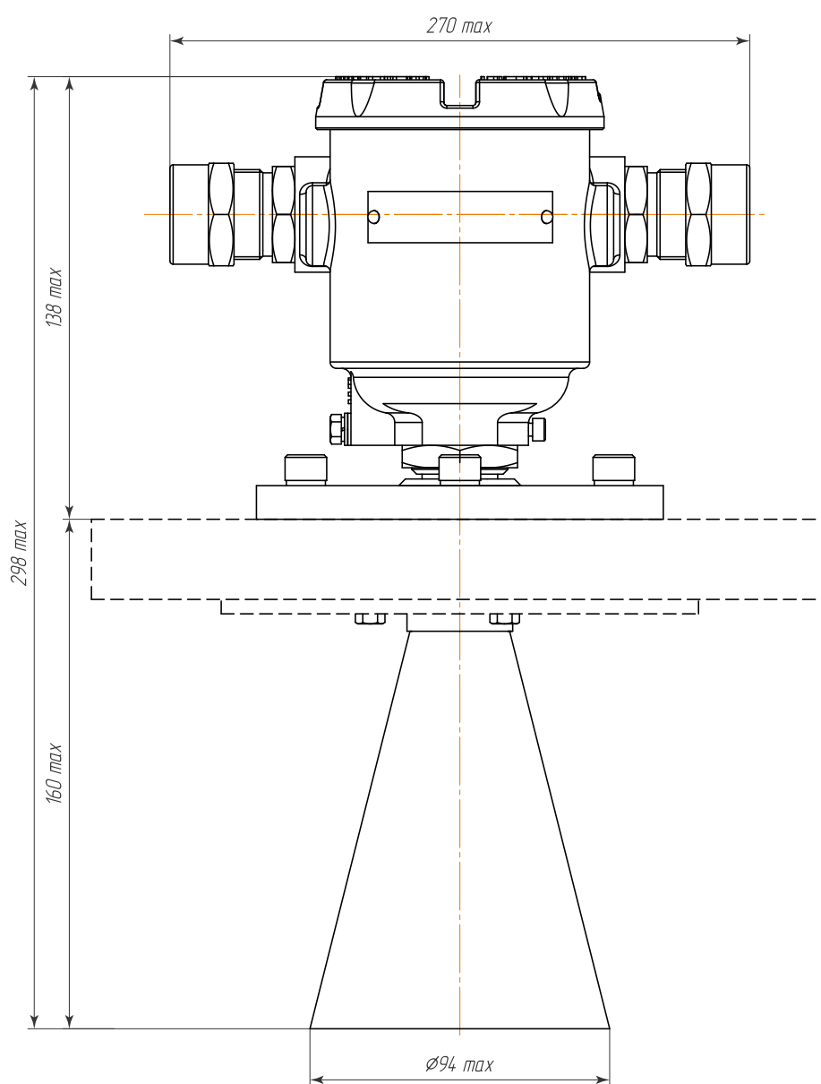
Уровнемер с базовым исполнением ABC
