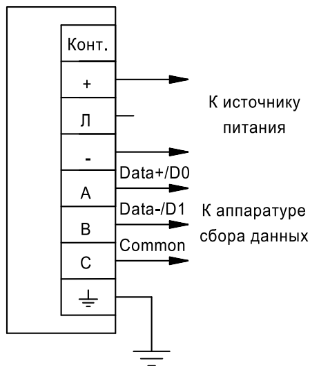
Схема подключения к системе с интерфейсом RS-485
