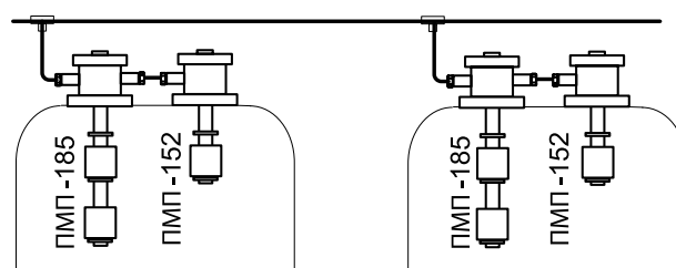
Дублирование самого себя датчиком ПМП-152 (ПМП-052)
