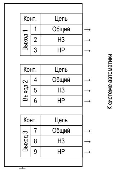
схема подключения выходов с переключающимся (П) состоянием
