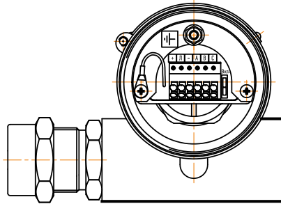
интерфейс RS-485
