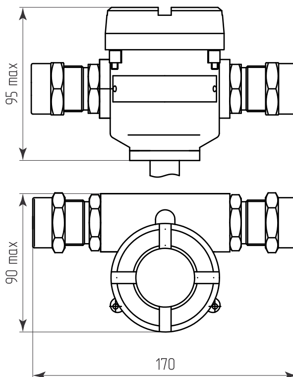
с двумя кабельными вводами
