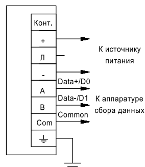
Схема подключения к системе с протоколом Modbus
