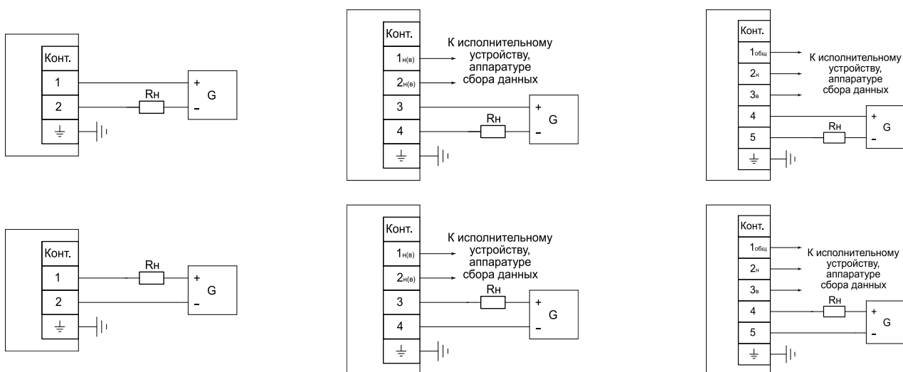
Схема подключения к интерфейсу 4-20 мА
