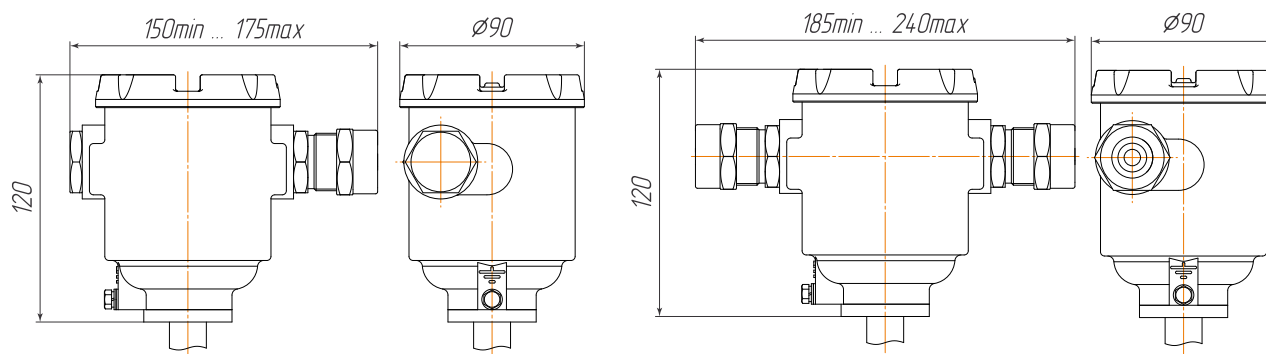
Корпус с одним кабельным вводом
