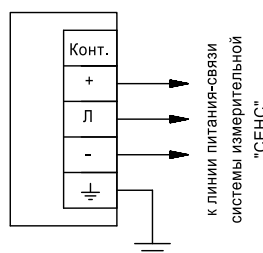
Схема подключения к системе с протоколом «СЕНС»
