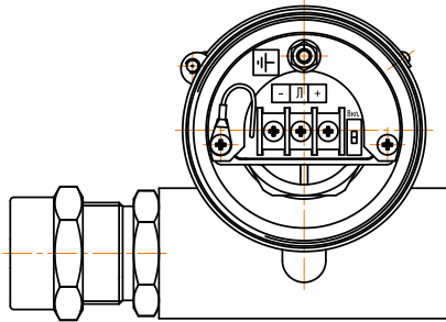
интерфейс СЕНС
