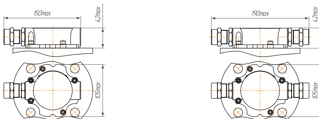
Литой низкопрофильный корпус с одним или двумя кабельными вводами D12
