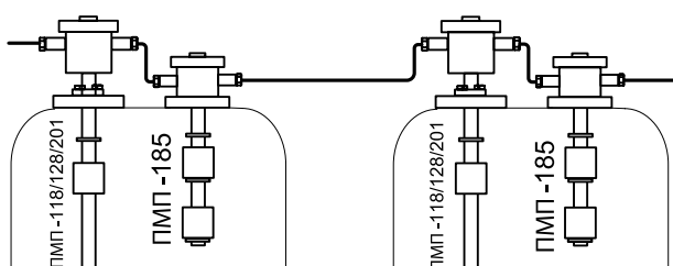
Дублирование уровнеймеров ПМП-118, ПМП-128, ПМП-201
