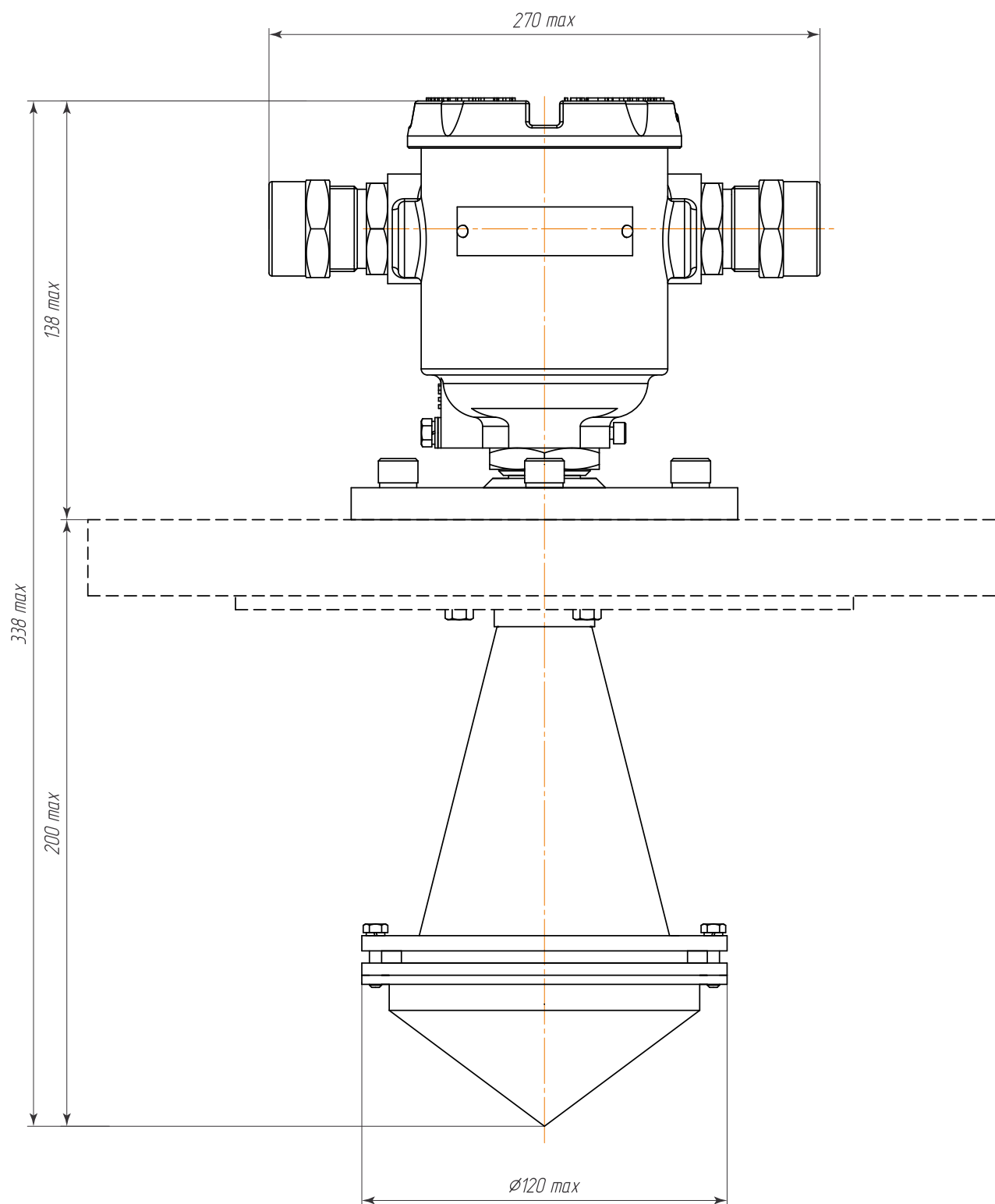
Уровнемер с герметизированной АВС
