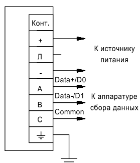
Схема подключения к системе с интерфейсом RS-485
