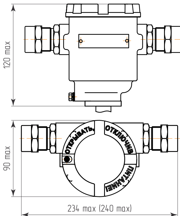
с двумя кабельными вводами
