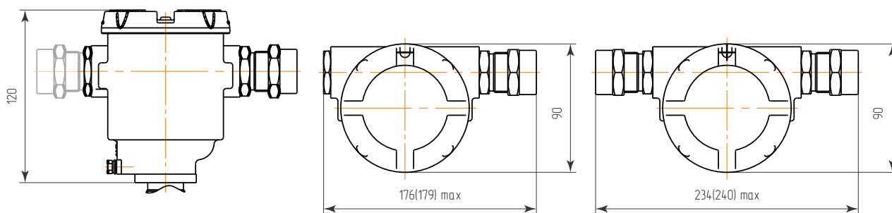
Литой корпус с одним или двумя кабельными вводами D12 (D18)
