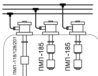
Тройное дублирование. Три преобразователя, отдельные линии и вторичные приборы
