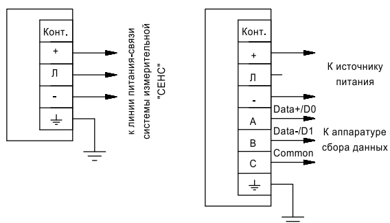
Схема подключения к системе с интерфейсом «СЕНС»
