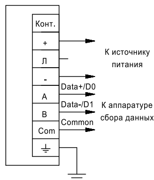
Схема подключения к системе с протоколом Modbus
