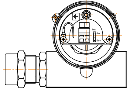
интерфейс 4/20 мА
