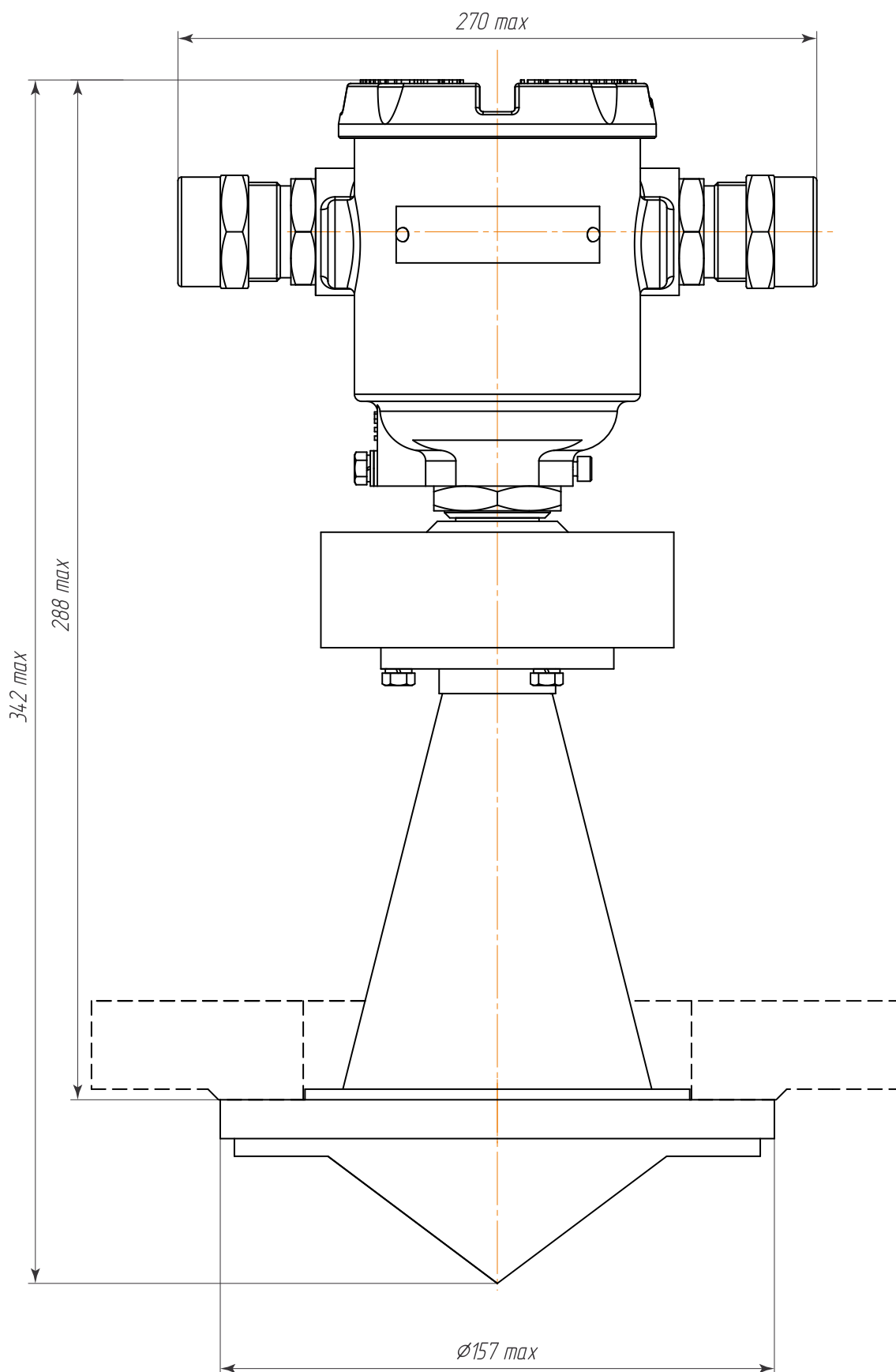
Уровнемер с изолированной АВС
