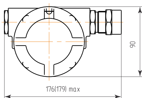
с одним кабельным вводом
