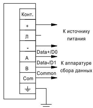
интерфейс RS-485
