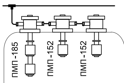
Тройное дублирование с ПМП-152 (ПМП-052)
