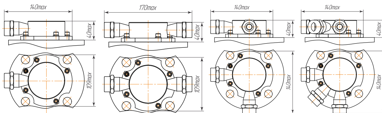
Сварной низкопрофильный корпус с одним, двумя или тремя приваренными кабельными вводами D12
