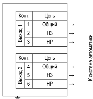
схема подключения выходов с переключающимся (П) состоянием
